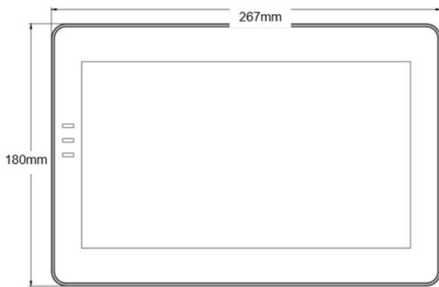
正面
